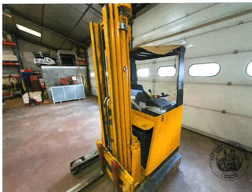
6. Transpalette Typ ETVA-12-GE-115-530 DZ N de série 773420604 3780 Heures
